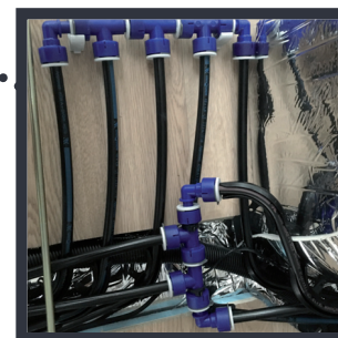
Réseau eau propre tuyaux semi-rigides raccord rapide avec centralisation nourrice de raccordement
