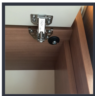
Support de fixation renforcé des meubles pavillons
